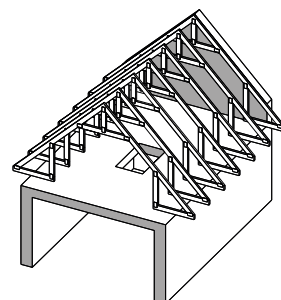
CHARPENTE EN FERMETTES POUR COMBLES HABITABLES (fig. 2)
