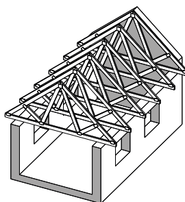
CHARPENTE EN FERMETTES POUR COMBLES PERDUS (fig. 1)
